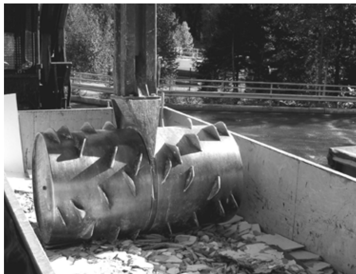
Kuvassa rullaava tela murskaa lastulevyä tiiviiksi paketiiksi
